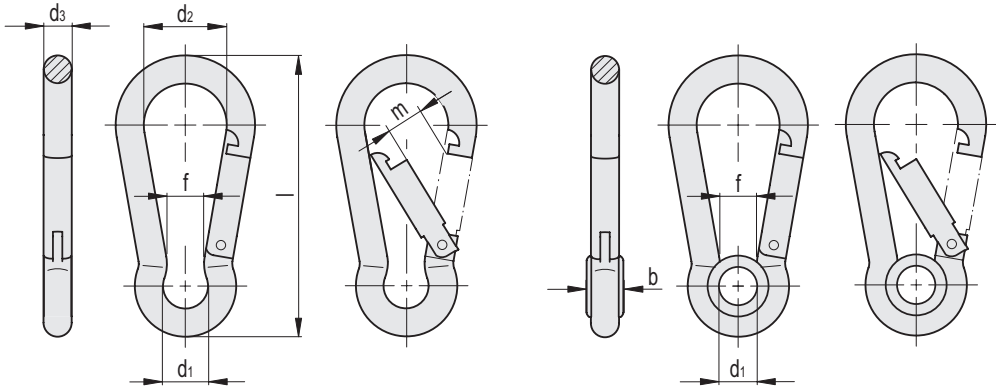
GN 5299-C-ST GN 5299-C-A4
